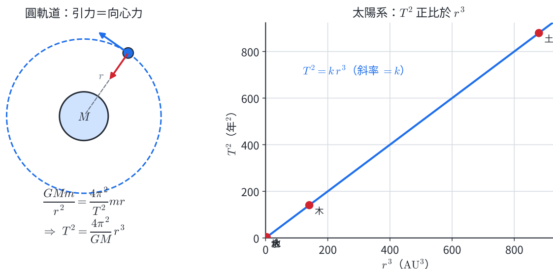
圖 6-5：左——由「圓軌道引力＝向心力」推得 T^2 = \frac{4\pi^2}{GM}r^3 。右——太陽系各行星的 T^2 對 r^3 作圖為一條過原點的直線，斜率為 k = \frac{4\pi^2}{GM} ，即 T^2 \propto r^3 。
