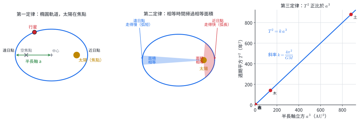
圖 6-4：克卜勒三大定律。左——第一定律：行星軌道為橢圓，太陽位於一個焦點（另一焦點為空），右頂點離太陽最近為近日點、左頂點最遠為遠日點。中——第二定律：行星與太陽連線在相等時間內掃過相等面積（兩塊陰影面積相等），故近日點走得快、遠日點走得慢。右——第三定律：太陽系各行星的 T^2 對 a^3 作圖為過原點的直線，斜率 k = \frac{4\pi^2}{GM} ，即 T^2 \propto a^3 。
